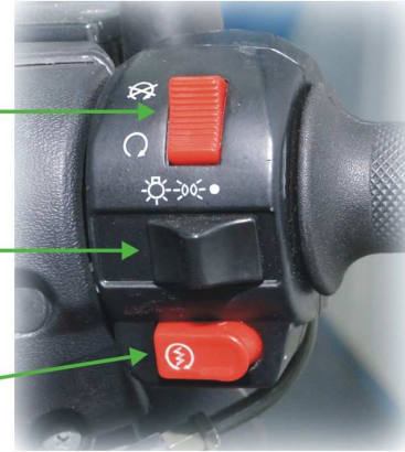
PRZEŁĄCZNIK ŚWIATEL POZYCYJNE / MIJANIA
